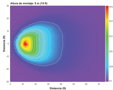
EM3-HI-MF - Luz proyectada media
