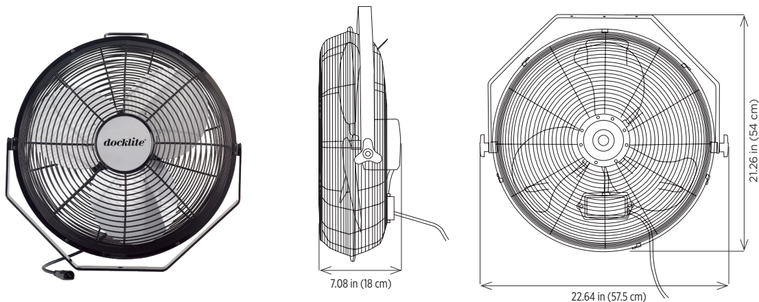
Fan DL-FAN-18
